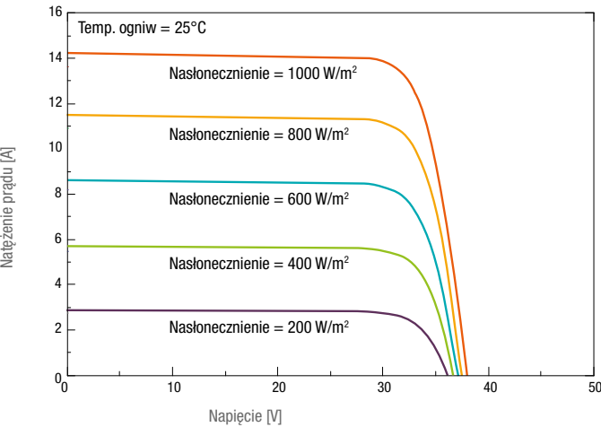
Krzywa prądowo/napięciowa modułu w zależności od nasłonecznienia
