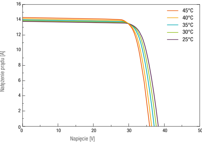
Krzywa prądowo/napięciowa modułu w zależności od temperatury
